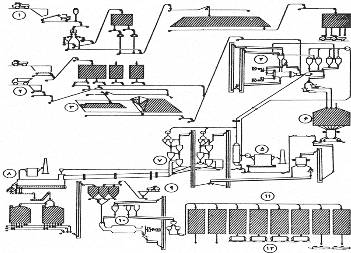
جانمای دستگاه‌های مختلف خط تولید سیمان
